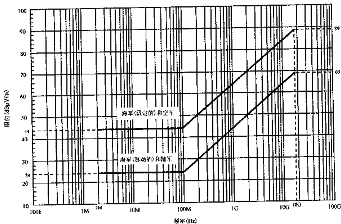
图 58 适用于地面的 RE102 限值
