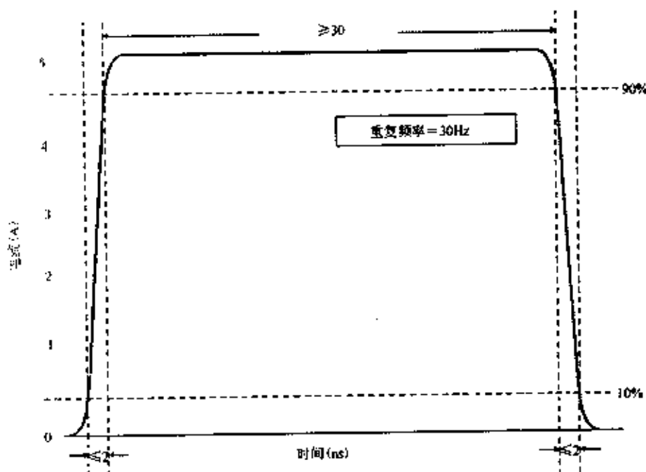
图 44 CS115 波形
