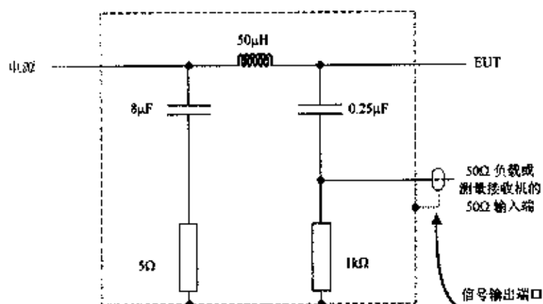
图6 LISN 电路图
