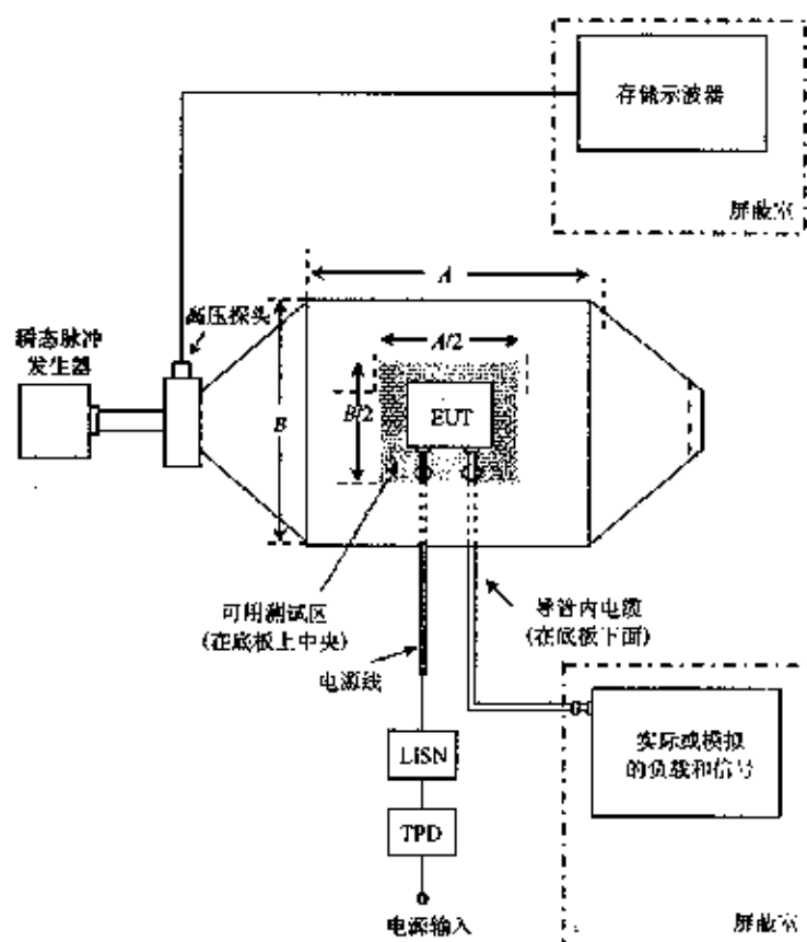
图 75 RS105 平行板辐射系统测试配置
