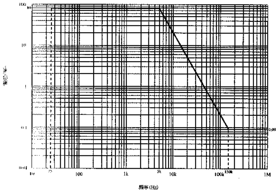
图 22 CS101 功率限值
