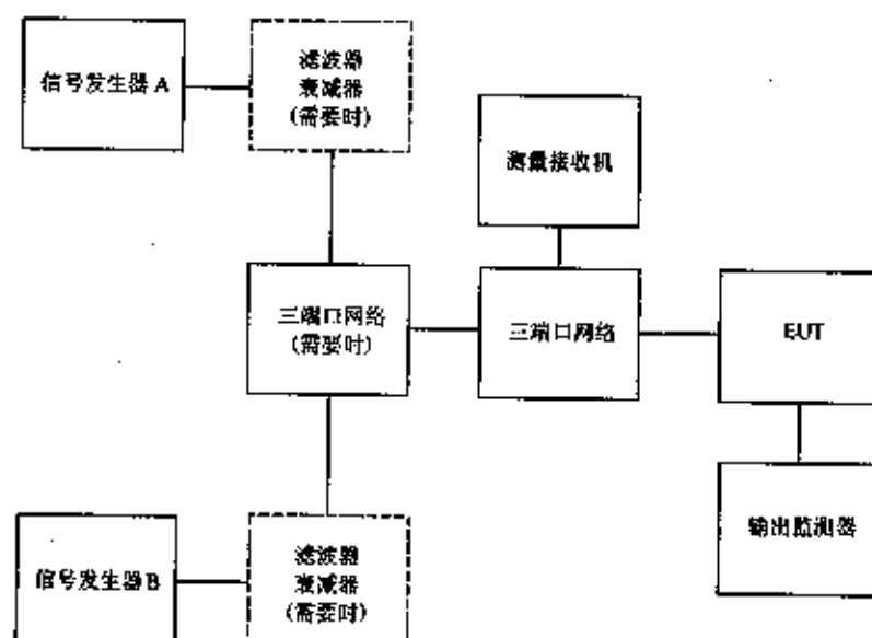
图 31 CS105 测试配置
