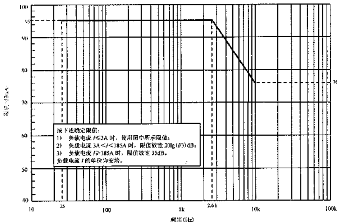
图 8 适用于潜艇的 CE101 限值(DC)
