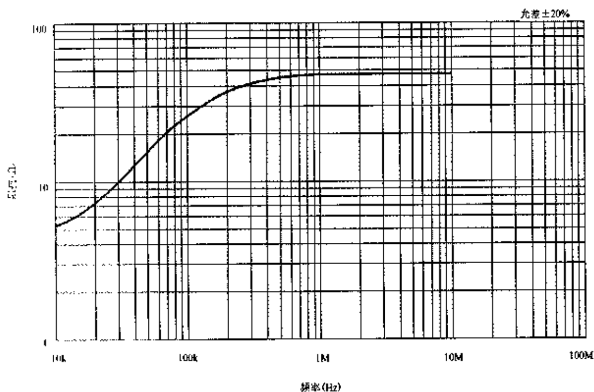
图7 LISN 阻抗
