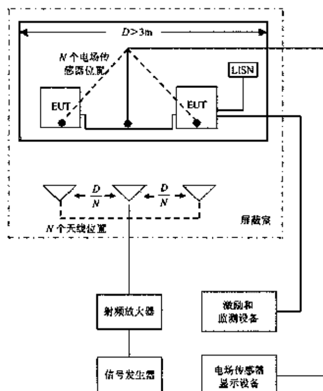
图 70 RS103 多天线布置(测试配置边界 D > 3\text{m} )
