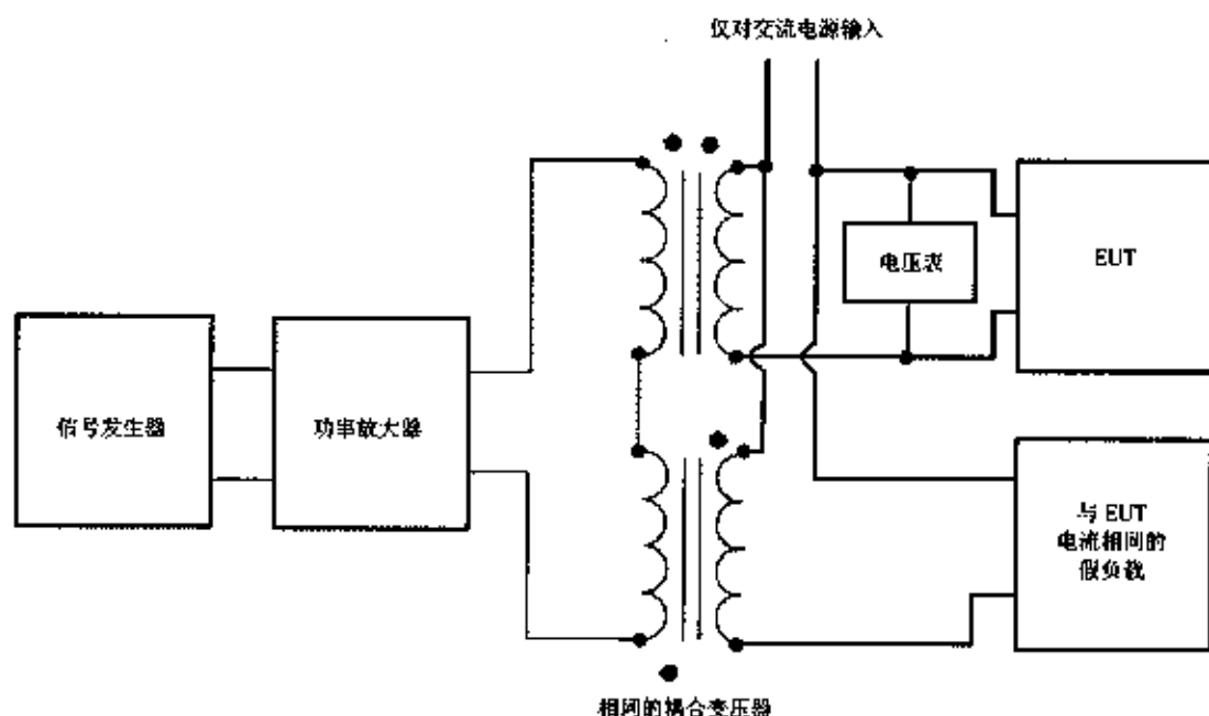
图 27 CS101 功放的保护
