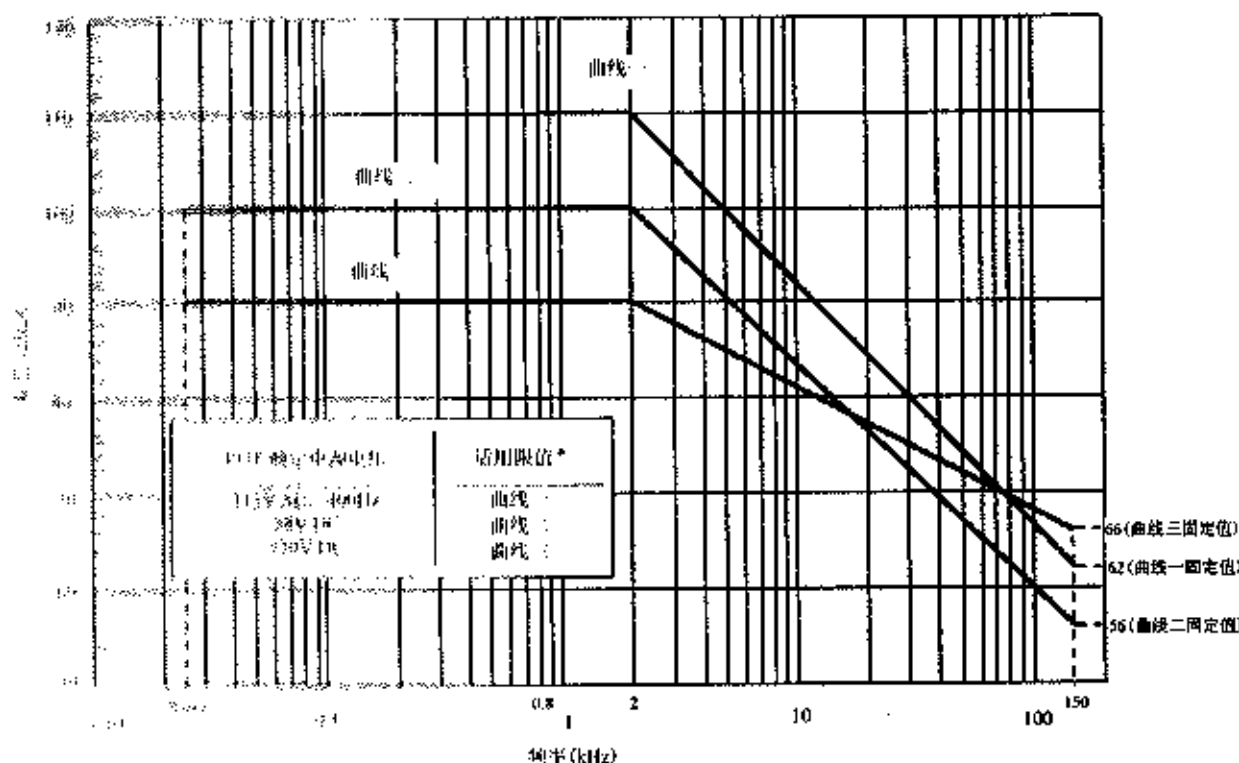
图 B.1 适用于 5\mu\text{H} LISN 的 CE101 限值
