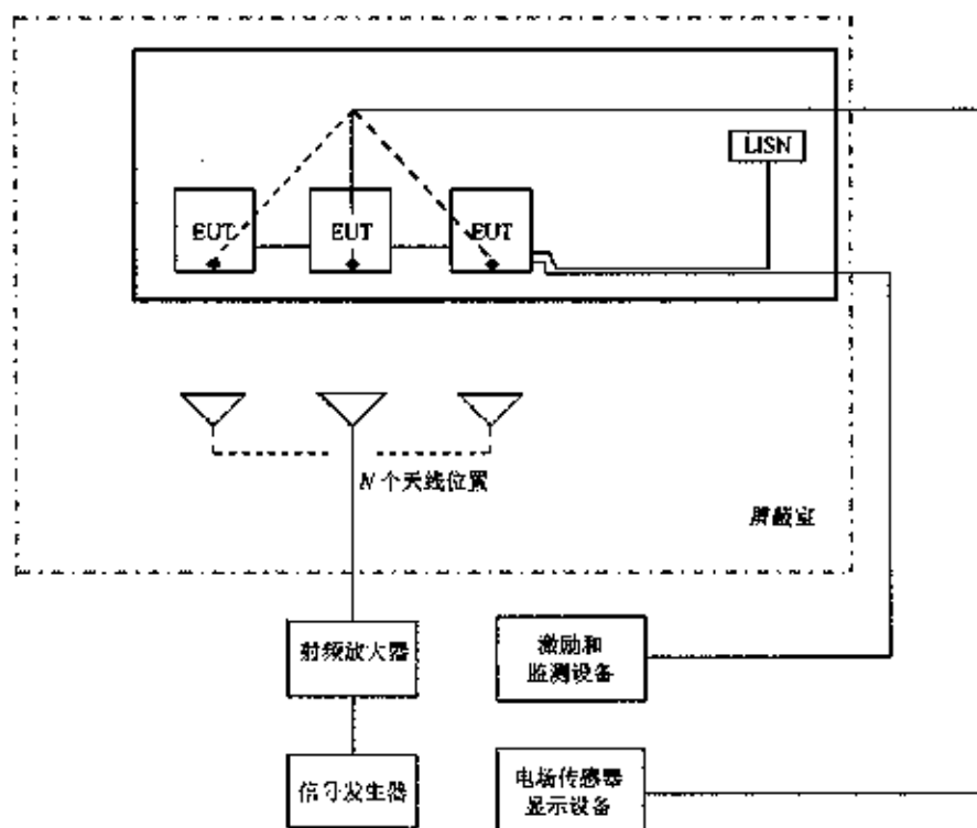
图 71 RS103 多天线布置( \geq 200\text{MHz} )
