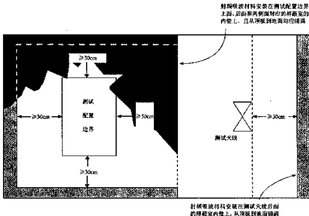
图 1 射频吸波材料安装图
