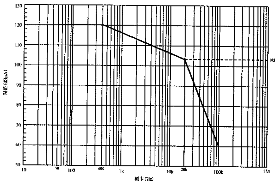
图 37 CS109 限值
