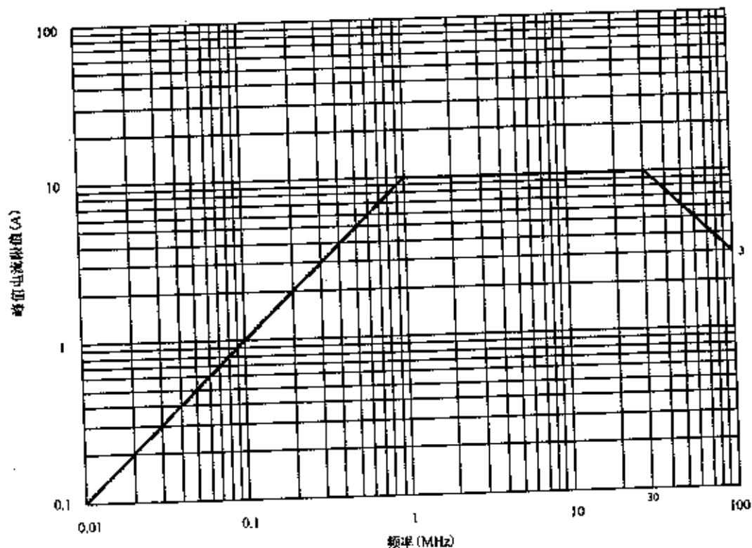
图 48 CS116 限值
